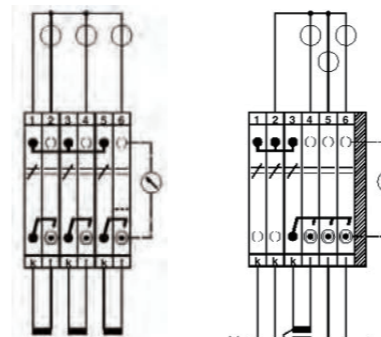
Пример подключения: Трехфазные трансформаторы тока
