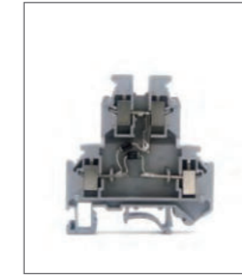
RUG/D-D Клемма с диодами Ширина 6.2мм / 0.5A / 4мм 2 Стр. 083
