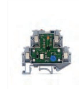
RUG-O-220AC/L/100mA Клемма с оптроном Ширина 6.2мм / 100mA / 4мм 2 Стр. 085
