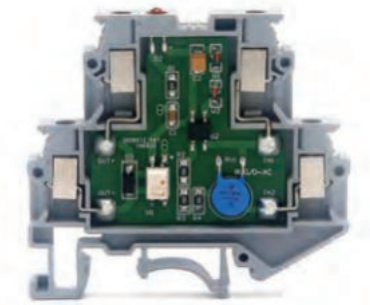
RUG-O-220AC/L/...mA
