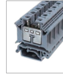
RUIK 16 Клемма универсальная Ширина 12.2мм / 101A / 16мм 2 Стр. 044
