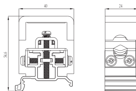
RMJ 2.5E
