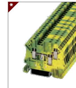
RUT 2,5-TWIN-PE Клемма универсальная заземляющая, 3 контакта Ширина 5.2мм / - А / 2.5мм 2 Стр. 034
