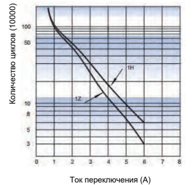
Электрическая долговечность
