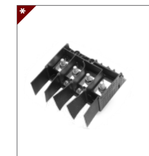
RBH 200A-4P Сильноточный клеммный блок с креплением на панель 1000В / 200А Стр. 164
