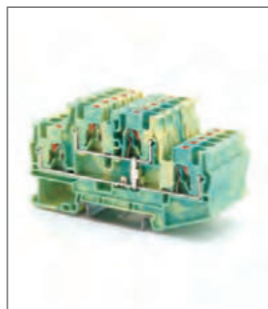
RPVTT 4-PE Клемма заземляющая, 3 уровня Ширина 6.2мм / - / 4мм 2 Стр. 024
