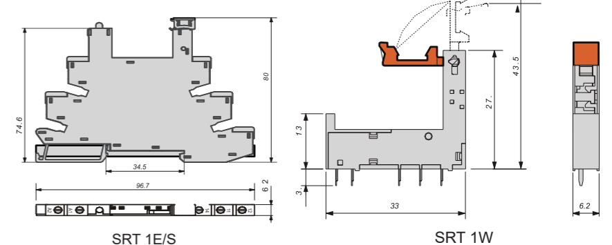
Габаритные размеры, установочный чертеж
