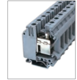
RUK 35N Клемма универсальная Ширина 15.2мм / 150A / 35мм 2 Стр. 045
