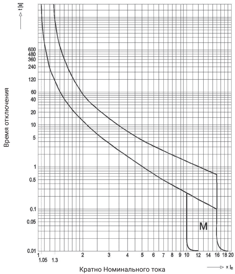
I_n > 10 \text{ A} Характеристики М EN 60 947-2
